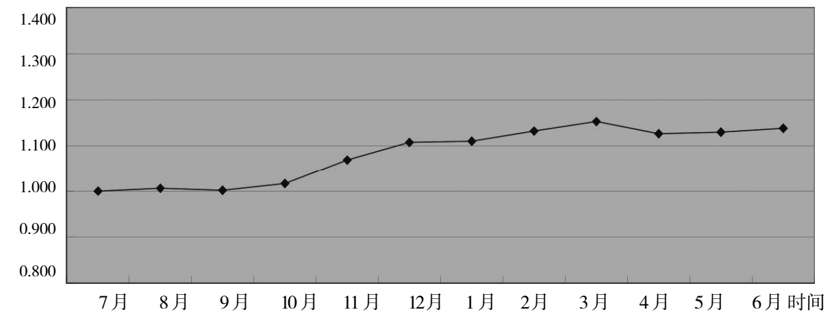
指数 2016年7月-2017年6月建设工程主材价格走势
