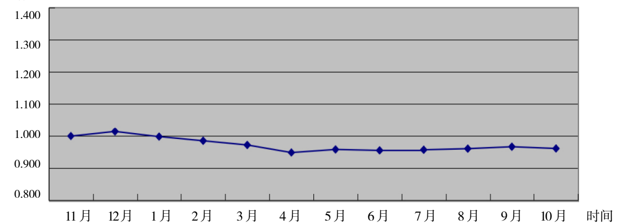
2019年11月-2020年10月建设工程主材价格走势
